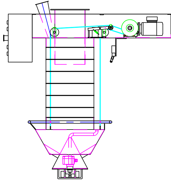
Abb. 2 Geschlossene Verladung - mit Aufsatzkonus (optional mit Drehflügelschalter) für Silofahrzeuge
