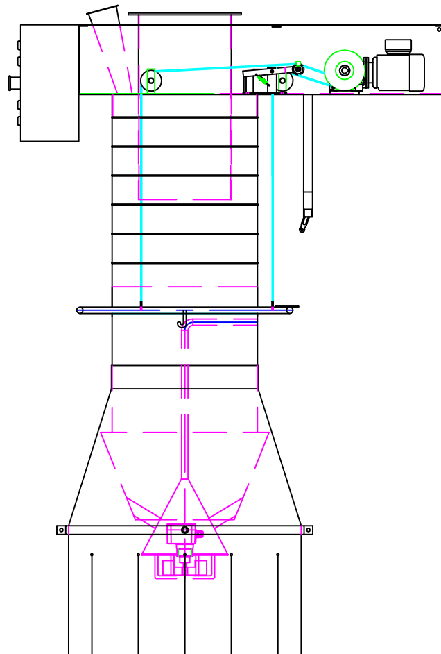
Abb. 3 Kombinierte Verladung - mit Aufsatzkonus und Auslaufglocke
