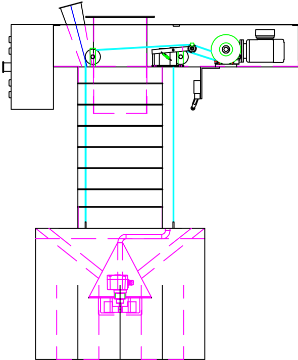
Abb. 1 Offene Verladung - mit Auslaufglocke (optional mit Drehflügelschalter) für Pritschenfahrzeuge
